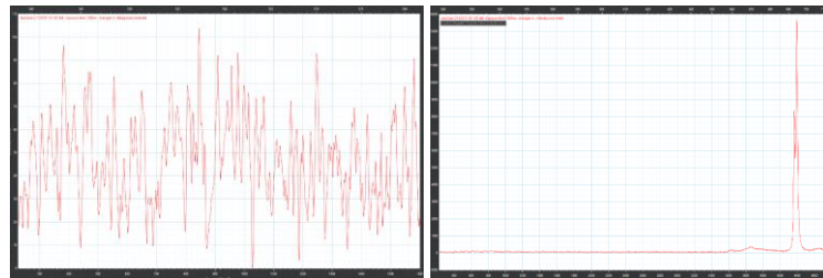
UV-vi s
