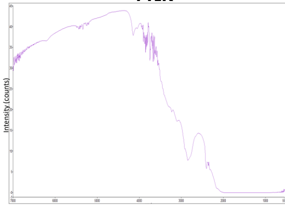
FTIR
