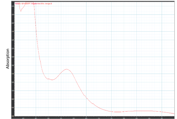
UV-vis
