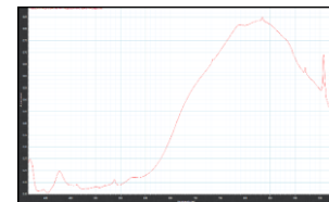
UV
