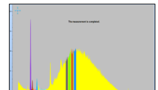
EDX
