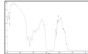
IR
