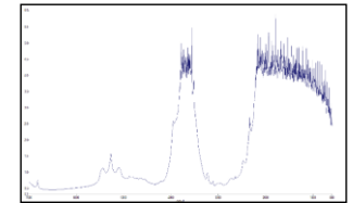
IR
